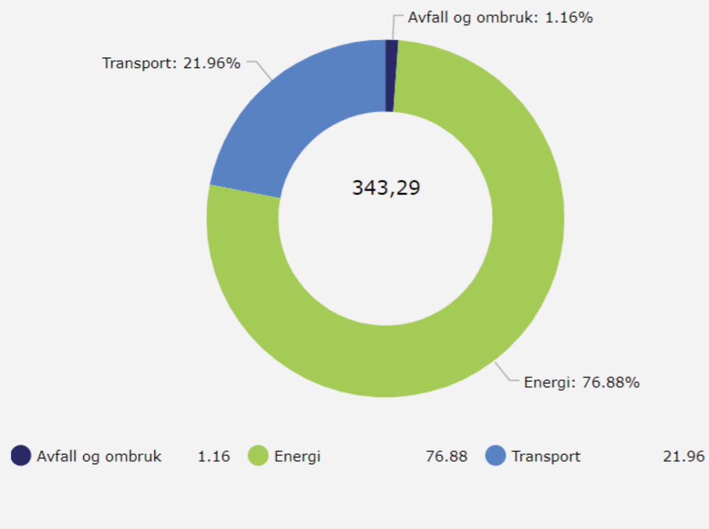
PROSENTVIS FORDELING AV CO2-UTSLIPP
