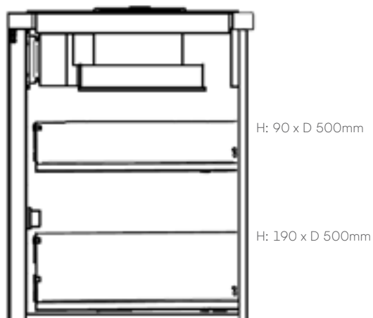
Standard seksjon for kullfilter (Bora)
