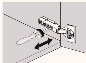
Justering dør inn/ut vertikalt
