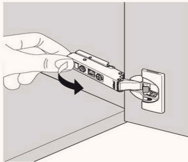
Demontering av dørhengsel fra festeplate
